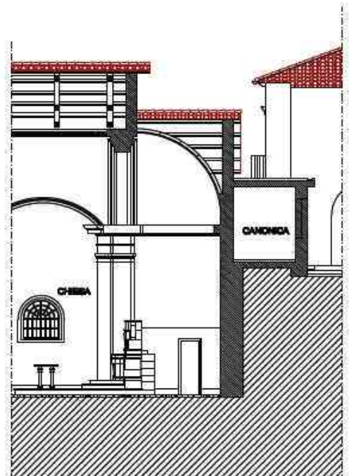
SEZIONE X - X
