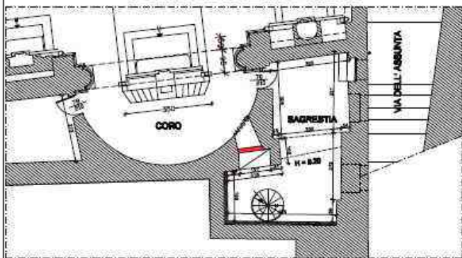
PIANTA PIANO TERRA - CHIESA
