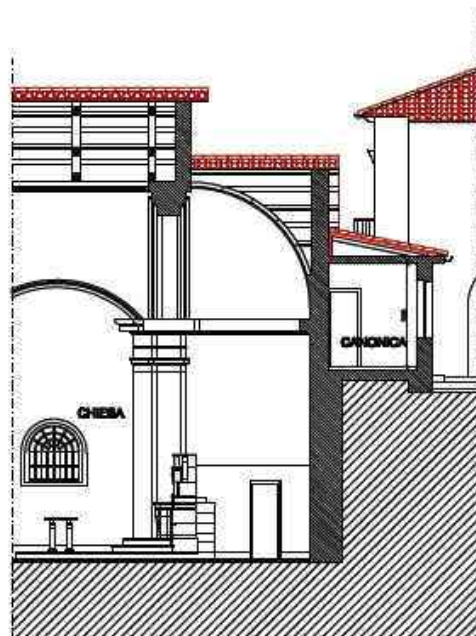
SEZIONE X - X
